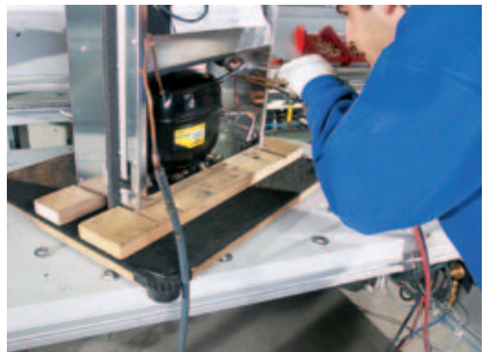
Sistema di montaggio manuale per la produzione di frigoriferi di fino a 75 kg di peso e a 2 m di altezza Sistema de montaje manual para la producción de equipos de refrigeración de hasta 75 kg de peso y 2 m de altura Sistema de montagem manual para a produção de refrigeradores com um peso de até 75 kg e altura de 2 m Pfannenberg GmbH, Hamburg, D Made by Handke Industrietechnik, Hamburg, D
